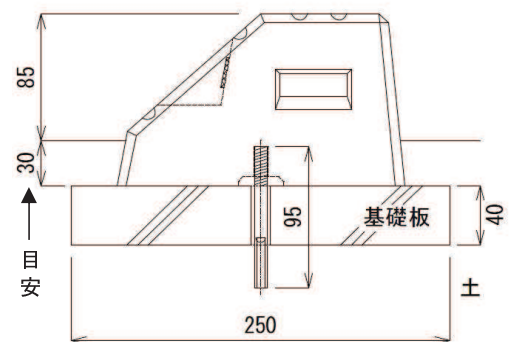
台付PB 設置状況(断面図)
